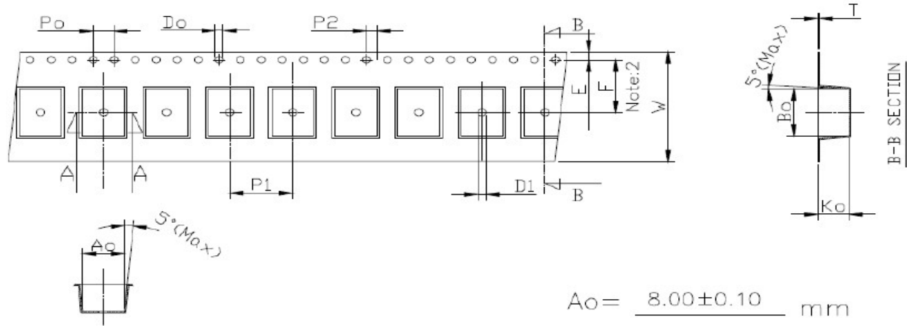
A-A SECTION
